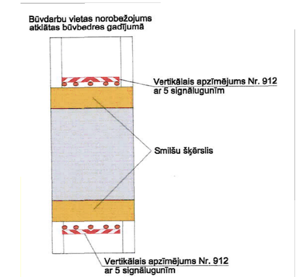
SATIKSMES ORGANIZĀCIJA DARBU VIETĀ - VARIANTS NR. 5
