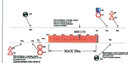
SATIKSMEŠ ORGANIZĀCIJA DARBU VIETĀ - VARIANTS NR. 1 (SLĒDZOT VIENU BRAUKŠANAS JOSLU)
