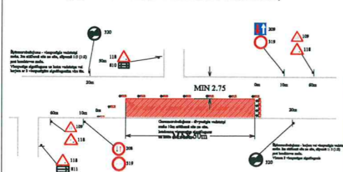
SATIKSMEŠ ORGANIZĀCIJA DARBU VIETĀ - VARIANTS NR. 2 (SLĒDZOT VIENU BRAUKŠANAS JOSLU)
