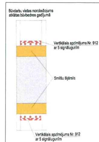
SATIKSMEŠ ORGANIZĀCIJA DARBU VIETĀ - VARIANTS NR. 3
